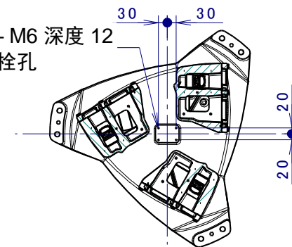
截面 C - C
