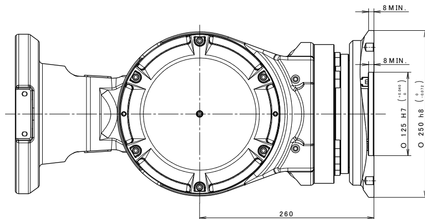
标准法兰
