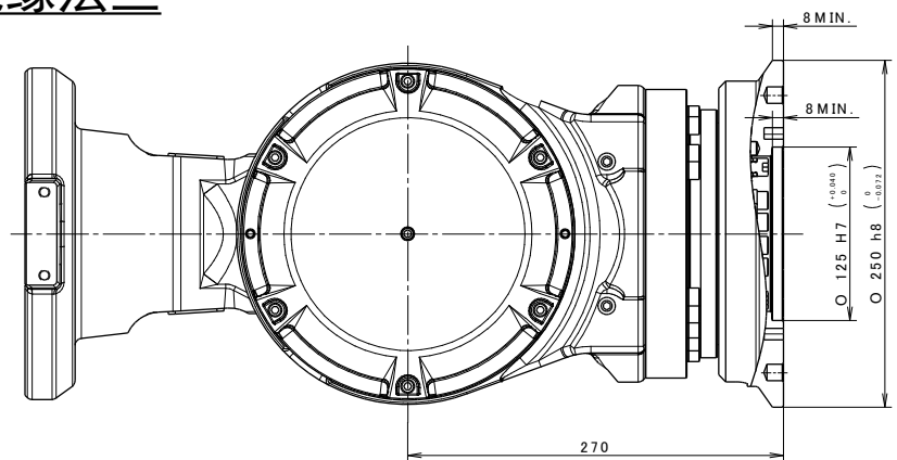
绝缘法兰
